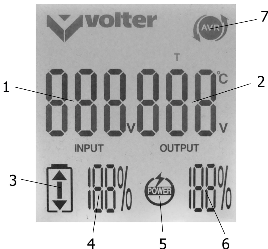
Рис.3. Жидкокристаллический индикатор
