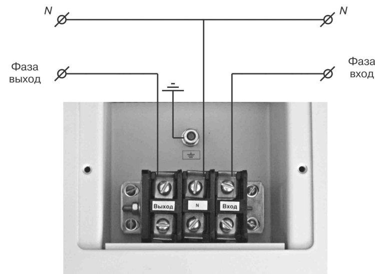
Рис. 4. Схема подключения стабилизатора
