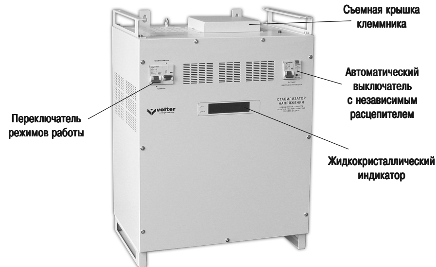
Рис. 1. Стабилизатор напряжения
