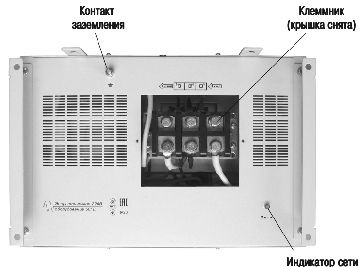
Рис. 4. Верхняя панель стабилизатора
